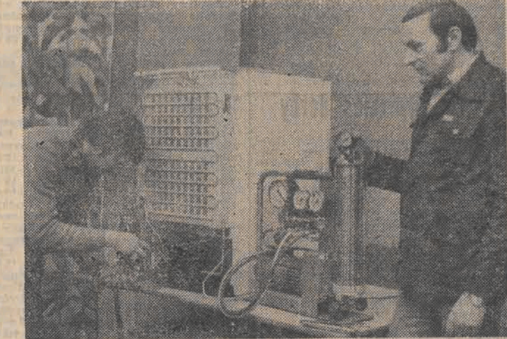
Witozak i Jan Wróblewski w czasie napełniania układu chłodzenia aparaturą „Refoco”.
