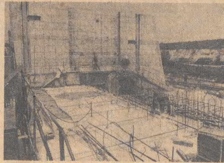
Na Wiśle, powyżej Krakowa, budowany jest stopień wodny „Kościuszko”, będący jedną z inwestycji zmierzających do całkowitej regulacji górnej Wisły. Budowa ma być zakończona w 1989 roku. CAF — M. Sochor
