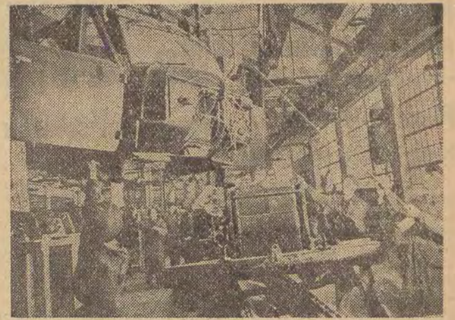
7 listopada z taśmy Fabryki Samochodów Ciężarowych w Lublinie zjechał pierwszy samochód „Lublin”. Na zdjęciu: Montaż naszego nowego samochodu ciężarowego przeprowadzają: Marian Kalita, Henryk Zaręba i majster Józef Kubica. (Patrz sprawozdanie z otwarcia na str. 2).
