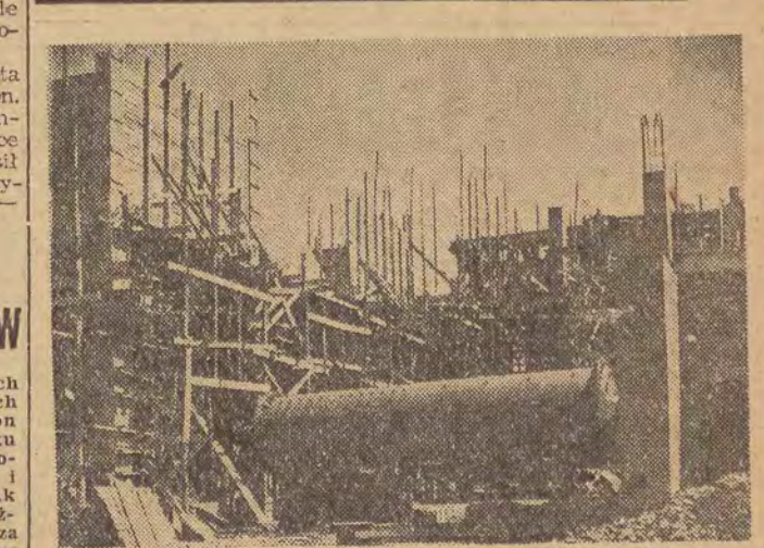
To zdjęcie przedstawia jeden z trzech tymnow kulowych, służących do rozdrabniania pyłu dymnicowych, gipsu i wapienia w budujących się przy ul. Wieniawskiego w Łodzi Zakładach Produkcji Elementów Budowlanych. Po uruchomieniu tej fabryki, w której wykorzystane będą najnowocześniejsze metody produkcji, łódzkie zagłębie budowlane otrzyma rocznie materiały budowlane w ilości ok. 100 milionów jednostek ceramicznych — tzw. piano-gazo-betonów.
