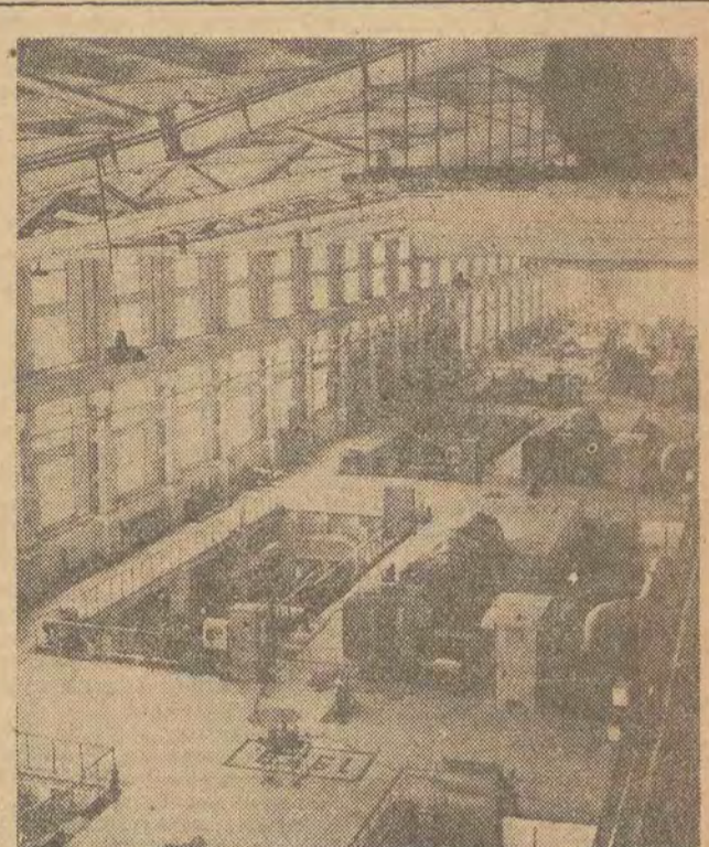
W tej oto hali (175 metrów długości) znajdują się turbozespoły. Jest ich w tej chwili pięć. Cztery już pracują, zaś piąty jest w fazie rozbudowy. Hala sprawi imponujące wrażenie. Zaledwie kilka osób obsługuje te olbrzymie maszyny. W przyszłości przewiduje się, iż cała obsługa składać się będzie zaledwie z 3 pracowników. O Łódzkiej Elektrociepłowni czytajcie na str. 3
