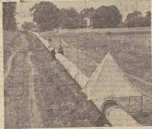
Przy budowie rurociągu naftowego w rejonie Plocka trwają przygotowania do opuszczenia odcinków rur do ziemi. Jedną z podstawowych prac — to spawanie. Ostatnio dzięki otrzymaniu nowoczesnej radzieckiej spawarki automatycznej tempo robót znacznie wzrosło. Oszczędność czasu jest ogromna, spawarka wykonuje jeden spaw w ciągu 5 minut, podczas gdy ręcznie praca ta trwała do 3 godzin. Na zdjęciu: spawanie rurociągu na trasie.
