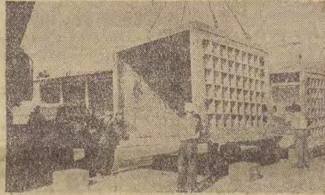
Na wystawie osiągnięć gospodarki ZSRR w Moskwie w dziale „Budownictwo” zademonstrowano nową technikę budowlaną. Na zdjęciu: instalowanie przy pomocy dźwigu elementu podziemnego kolektora przechodzącego sporządzonego z płyt wibro-wanych. Fot. — CAF
