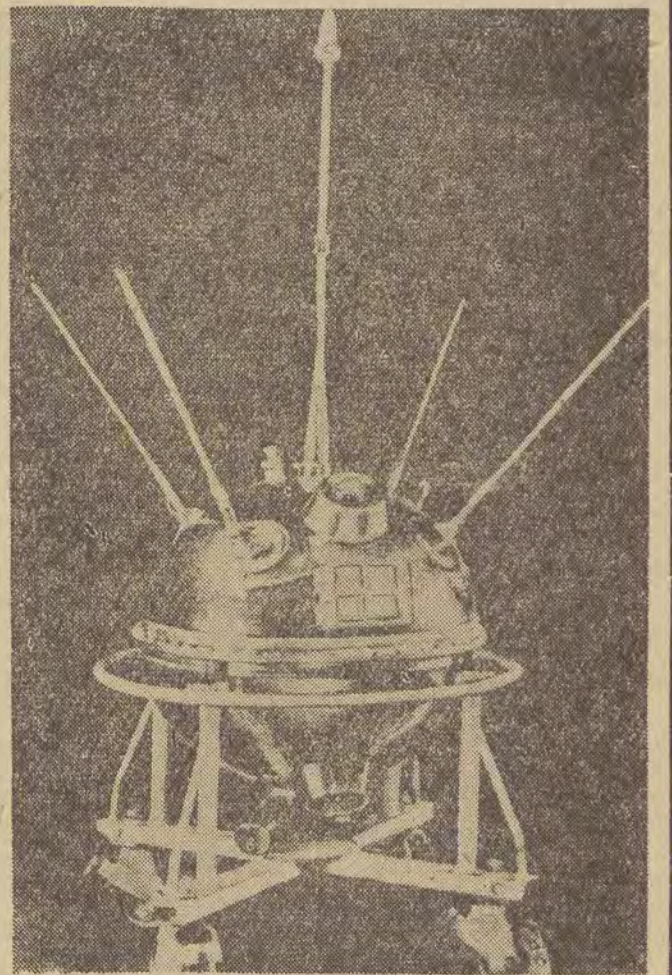
Radziecka rakietka kosmiczna. Pojemnik z aparaturą naukową i pomiarową podczas montażu.
