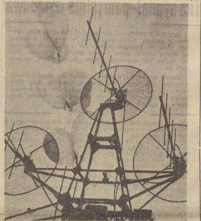
Badania wyższych warstw atmosfery prowadzone są w ZSRR przy pomocy specjalnych rakiet, wystrzeliwanych ze stacji aerologicznych na terenie Związku Radzieckiego, oraz z pokładu statków, przeprowadzających obserwacje meteorologiczne. Na zdjęciu: urządzenia radiolokacyjne do śledzenia lotu rakiet meteorologicznych. FOT — CAF
