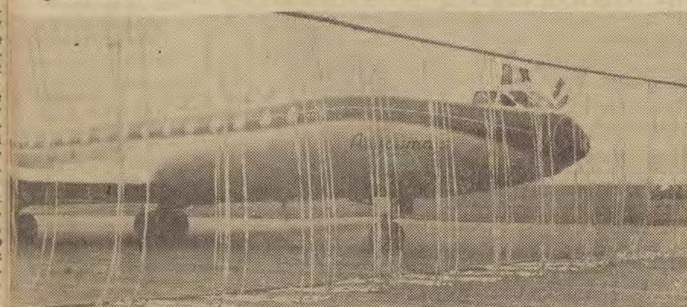
Naukowcy francuscy opracowali nowy system zatrzymywania samolotów na lotniskach z zbyt krótkim pasem startowym. Polega on na włączeniu przy pomocy fotokomórki specjalnego urządzenia złożonego z mocnych, nylonowych pasów. Pasy te powstrzymują samolot jeśli na końcu pasa startowego ma on jeszcze zbyt wielką szybkość. Specjaliści sądzą, że nowe urządzenie zmniejszy poważnie niebezpieczeństwo katastrof. Na zdjęciu: francuski samolot wojskowy przed nylonową barierą.
