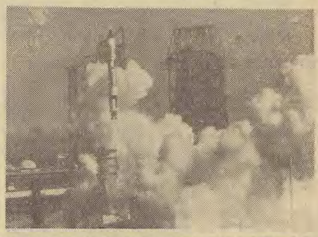
Na zdjęciu: start rakiety nośnej Titan-2 z umieszczonym na jej szczycie statkiem „Gemini-5”. CAF - Photofax
