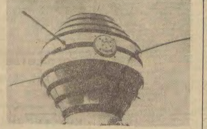
W ostatnich dniach listopada z poligonu rakietowego Hammaguir na Saharze ma zostać wystrzelona 30 rakiet typu „Diamant”, która wyniesie na orbitę okołoziemską pierwszego francuskiego sztucznego satelity „A-1”. Na zdjęciu: „A-1” o wadze 40 kg, średnicy 50 cm. CAF — Photofax
