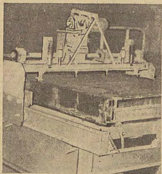
Wczoraj, w Łódzkich Zakładach Produkcji Elementów Budowlanych (Wieniawskiego 5) uruchomiono — drugie w Polsce — automatyczne urządzenie do ścinania nadrostów elementów. Zastosowanie tego urządzenia pozwala podnieść jakość produkcji i obniżyć znacznie jej koszt. Dotychczas prace te wykonywano ręcznie.
