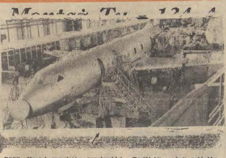
ZSRR. Montaż samolotów pasażerskich „Tu-134A” w hali zakładów lotniczych w Charkowie. CAF — TASS
