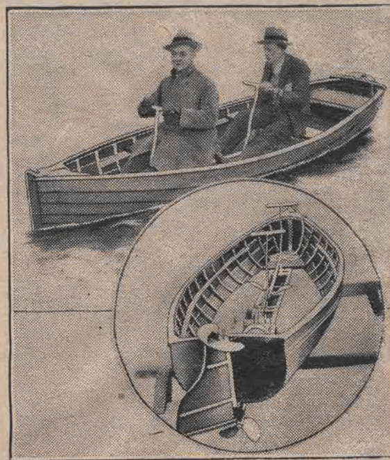
Nowy model łodzi, poruszanej sposobem pedałowym i zaopatrzonej w śmigło przy sterze.
