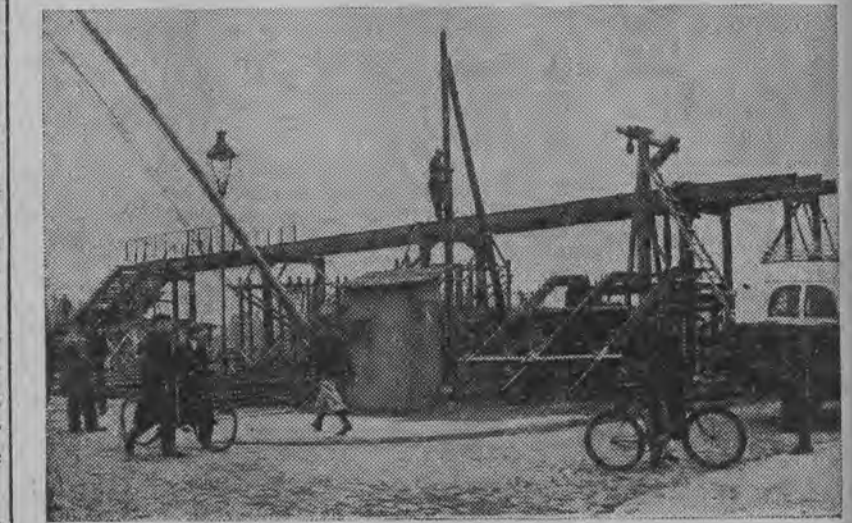
Montaż kładki nad torem przy ulicy Srebrzyńskiej
