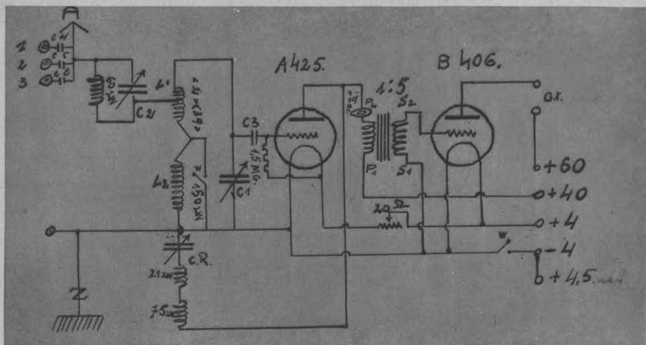
Schemat odbiornika dwulampowego (patrz artykuł w dzisiejszym „Głosie Porannym“).
