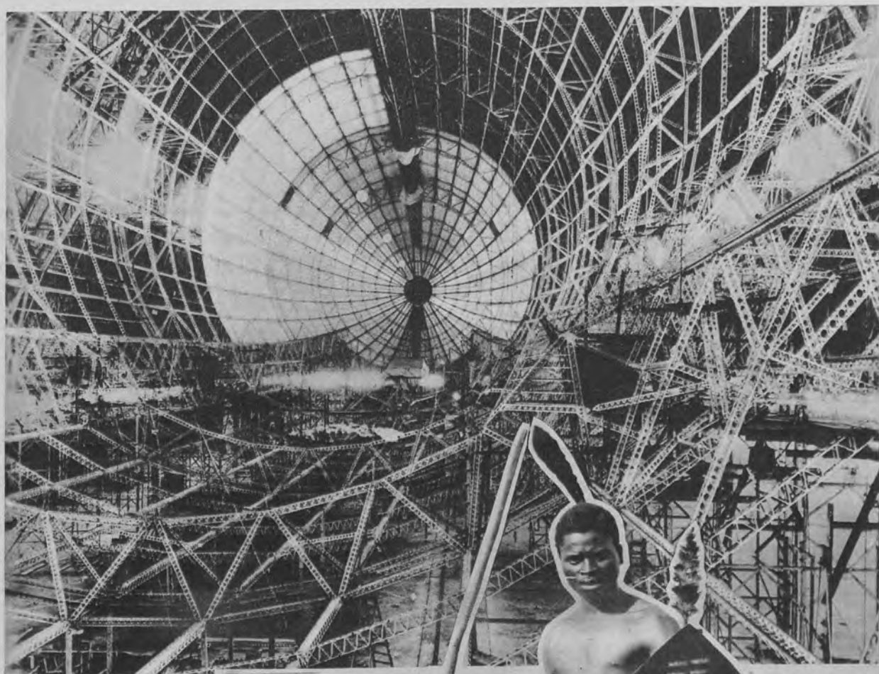
Szkielet olbrzyma sterowca budowanego na wzór Zeppelina w am. warsztatach w Akron (Stany Z. A.)
