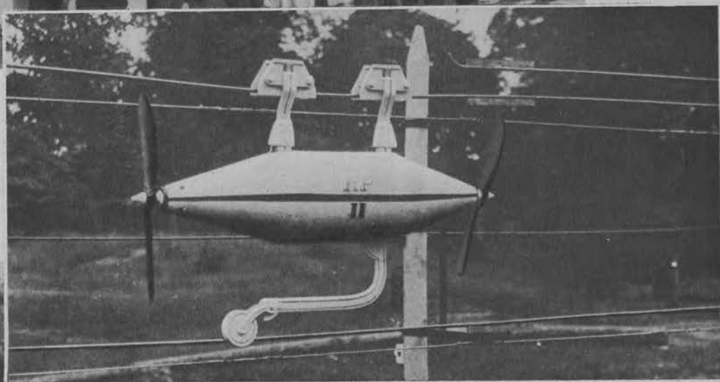
Na prawo: Próbna rakietka pocztowa zbudowa- na przez inż. Ryszarda Pfautza. Praktyka wykaże czy będzie ją moż- na zastosować na wielkie odległości.
