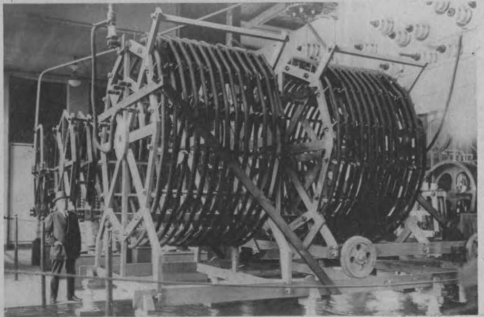
Gigantyczne urządzenie stacji radiowej w Nauen.
