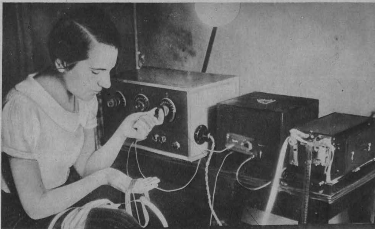
Niemiecka poczta wprowadziła między Berlinem a Hamburgiem aparaty radiowe do użytku handlowców nadające i odbierające listy. Odbieranie nadawanego listu.
