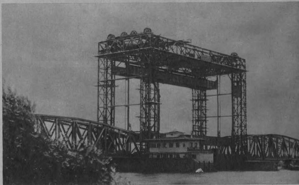
Most w Swinoujściu, którego środkowa część — dla przepuszczania statków — może być podnoszona 34m. nad poziom wody.
