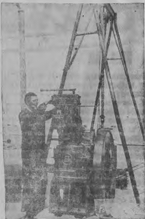
Montowanie maszyny.
