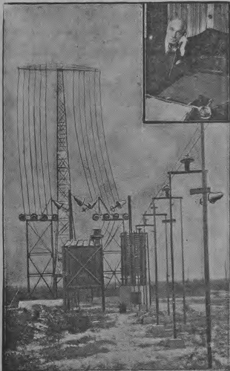
Anteny stacji radiotelegraficznej w Rocky-Point pod Nowym Jorkiem. W rogu poseł amerykański w Berlinie.
