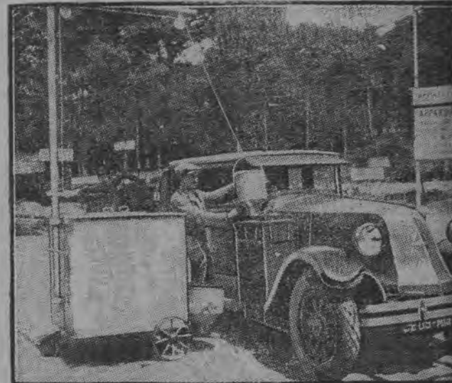
40-konny samochód, poruszany gazem drzewnym. zaopatrywania w węgiel drzewny.
