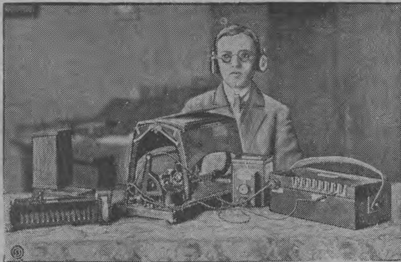
Angielski fizyk, Fournica d'Albe, skonstruował aparat, nazwany przezeń „Optofonem”, umożliwiający ślepcom czytanie każdej książki. Na naszej fotografii czytana książka leży na aparacie, który fale świetlne przetwarza na słuchowe.
