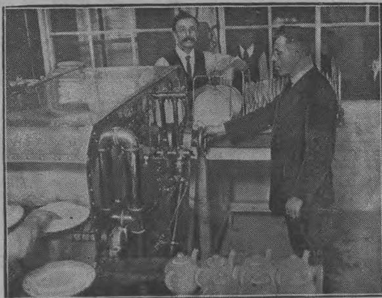
Maszyna do mycia naczyń stołowych, pracująca w jednym z wielkich hoteli londyńskich.
