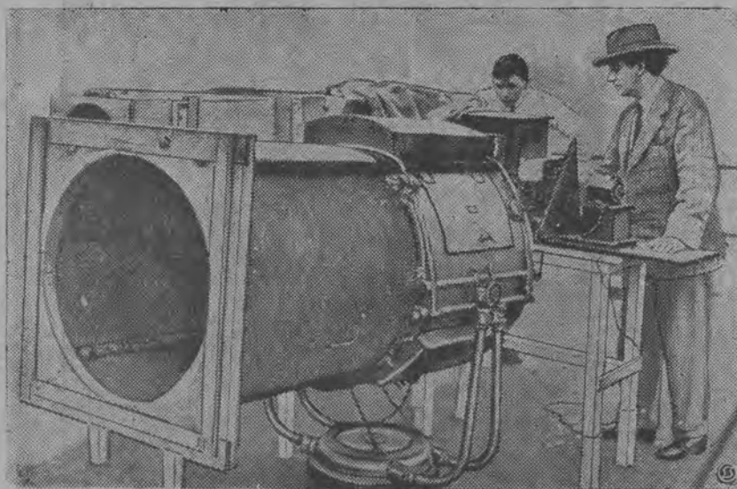
„Noctevisor”, aparat, wynaleziony przez Anglika Bairda. Aparat ten pozwala rozróżniać przedmioty w nocy nawet podczas mgły.
