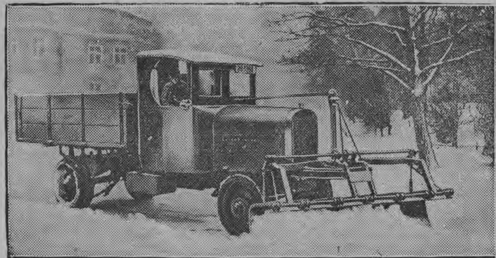
Samochód do zgarniania śniegu, zastosowany ostatnio na ulicach Berlina.
