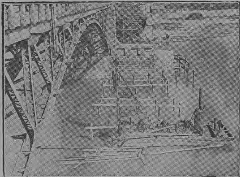
Po odbudowaniu „półmościa” Poniatowskiego, obecnie przystąpiono do odbudowy pierwszego przęsła na całej szerokości.
