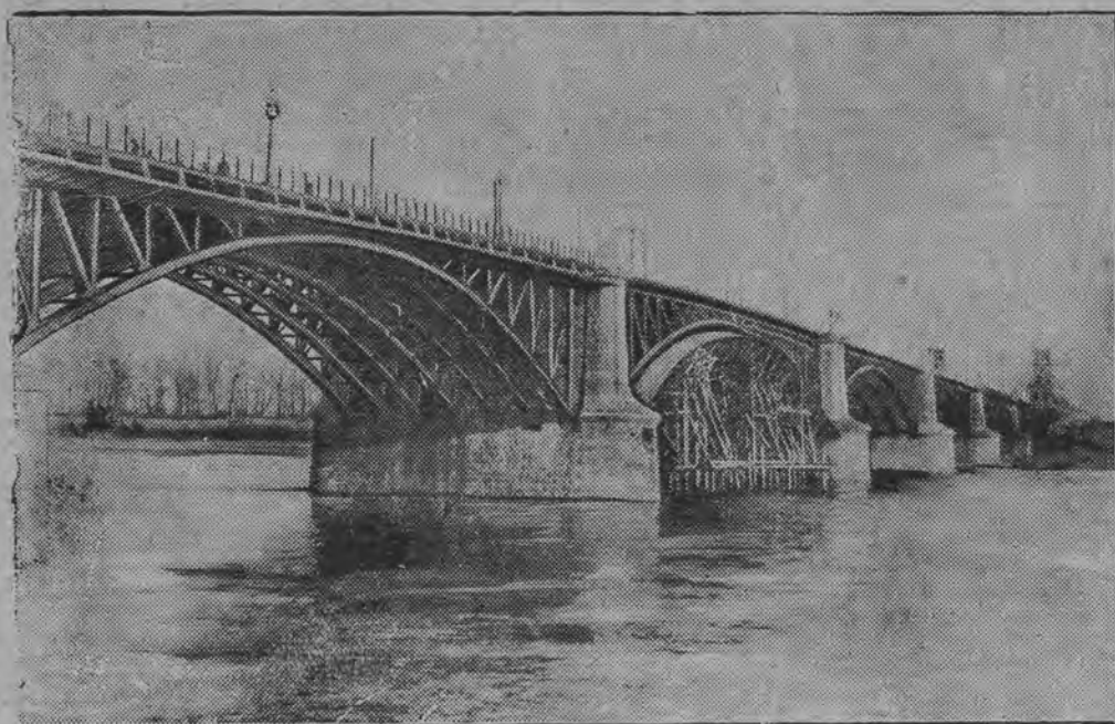
Widok zmontowanych przęseł drugiej połowy mostu Poniatowskiego.
