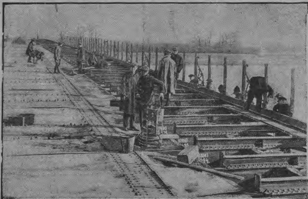
Ostatnie roboty przy montażu 4 go przęsła.
