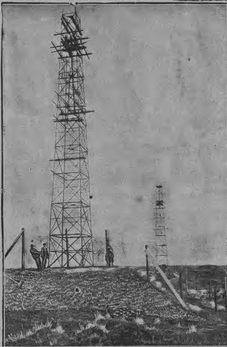
Strzeliste anteny budowanej w Mokotowie nowej stacji nadaw- czej radjotelefonicznej są już na ukończeniu.
