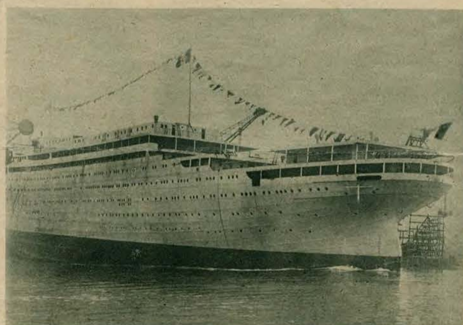
W Monfalcone pod Triestem, wykończono i spuszczone na morze największy na świecie okręt motorowy. Mierzy on 193 metrów długości, 25 szerokości i z powodu wielkiej ekonomii miejsca, osiągniętej dzięki brakowi kotłów, pomieścić może 3.000 pasażerów i 10.000 ton towaru. Motory tego okrętu, rozwinąć mogą siłę 35.500 koni.
