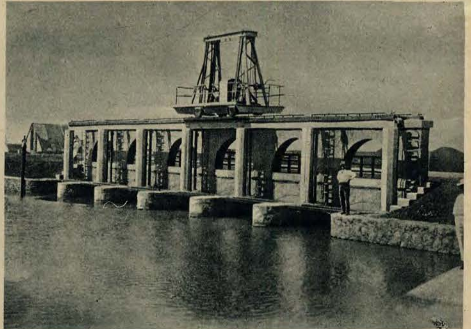
W tych dniach poświęcono nową tamę na Niebieskim Nilu, która jest cudem nowoczesnej techniki. Długości około 3 km., użyłnia 312.000 akrów ziemi, a koszt wynosił ok. pół miliona złotych. Na zdjęciu widoczna jedna z licznych śluz tamy.
