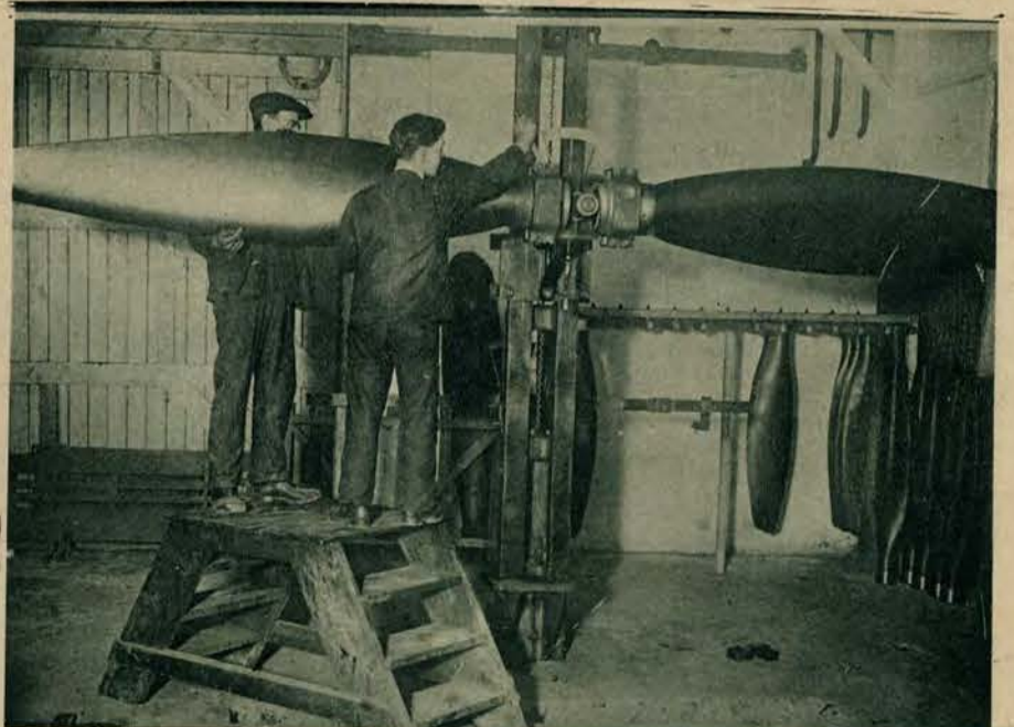
Największa śmigła (propeler) świata zbudowana jest z płyt stalowych i, będąc w środku próżna, jest znacznie lżejsza niż śmigła drewniana tych samych wymiarów. Jest angielskiej konstrukcji i przeznaczona do balonu R. 101.
