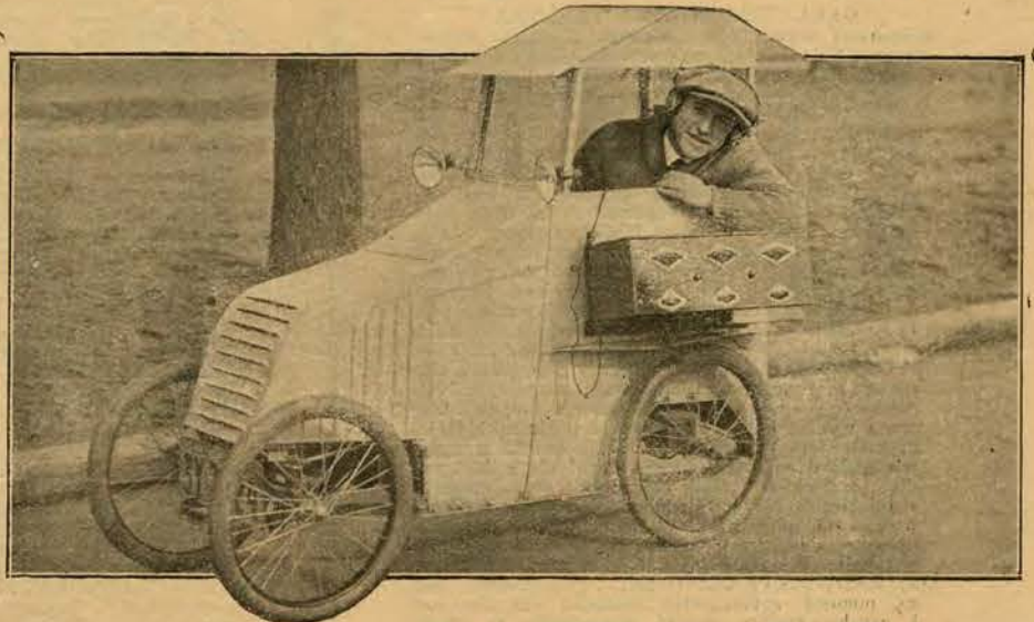
Najmniejszy samochód, wykonany w przeciągu 9 miesięcy przez Izydora Lubin'a w Brooklynie. Posiada jeden cylinder, waży 150 funtów, rozwija szybkość 65 klm. na godzinę i zaopatrzony jest w radio-odbiornik.
