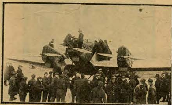
Dnia 24 lutego odleciał do Angory w Turcji Azjatyckiej samolot typu Junkersa zbudowany w fabryce A. B. Słygindystry w Linhann z metalu i posiadający trzy silniki o sile 900 koni a skrzydła o rozpiętości 28 i pół metra. Waga samolotu wynosi 3600 kg a z ładunkiem i pasażerami 6000 kg. Zdjęcie nasze przedstawia samolot na lotnisku Mokotowskiem przed odlotem.
