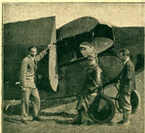
1) Awionetka polska „K.W.D. 3”. 2) Maszyna K.W.D. 3”, mająca składane skrzydła, wykonana przez studentów politechniki warszawskiej.
