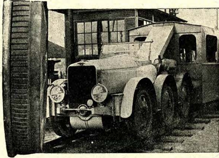
Dokonano we Francji ciekawej próby — zastosowania opon gumowych do sprzętu kolejowego o napędzie benzynowym. Próby dały znakomity wynik, przyczem stwierdzono, że 300-konny silnik daje możliwość rozwinięcia szybkości 140 klm. na godzinę.
