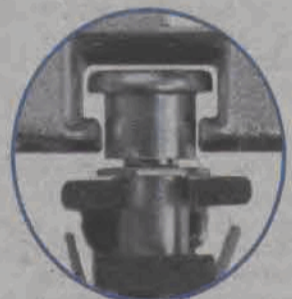
Czop i.S. wraz z zaczepem antywyważeniowym Safety Plus
