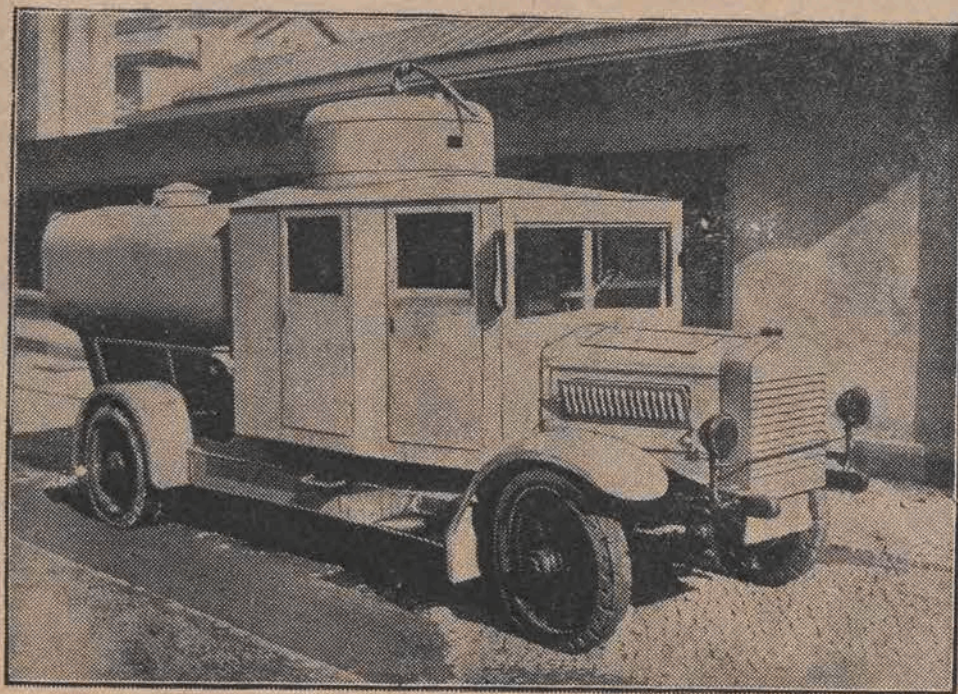
Policja berlińska została wyposażona w samochód - sikawkę do roz- pędzania tłumów. W zbiorniku mieści się 5000 litrów wody. Pompa jest tak silna, że może wyrzucić strumień wody na 50 mtr. Samochód ten wy- kazał już swą dużą użyteczność praktyczną.
