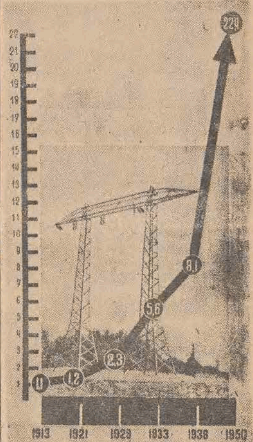
Poleźny wzrost produkcji elektrycznej (moc elektrowni w milionach kilowatów)
