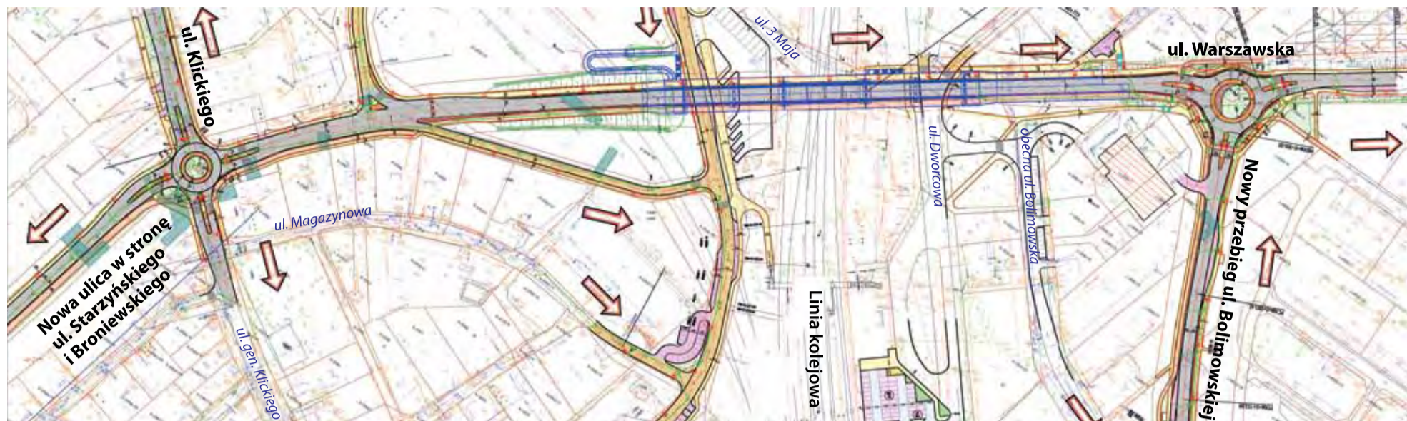
Projekt wiaduktu drogowego nad linią kolejową z projektowanym układem drogowym w Łowiczu
