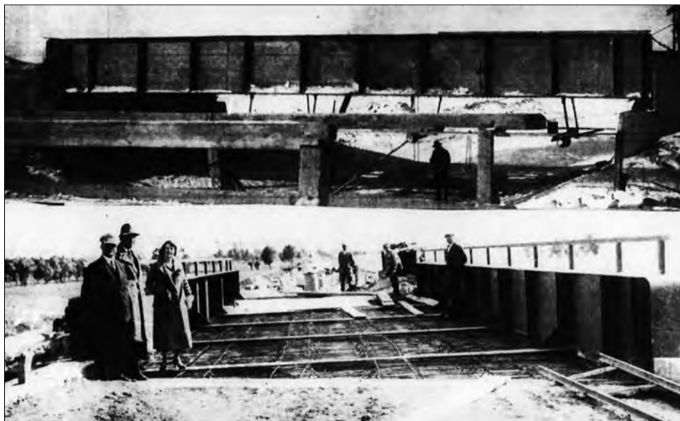
Budowa drugiego mostu spawanego na rzece Słudwi, fot. z 1931r., ze zbiorów autora
