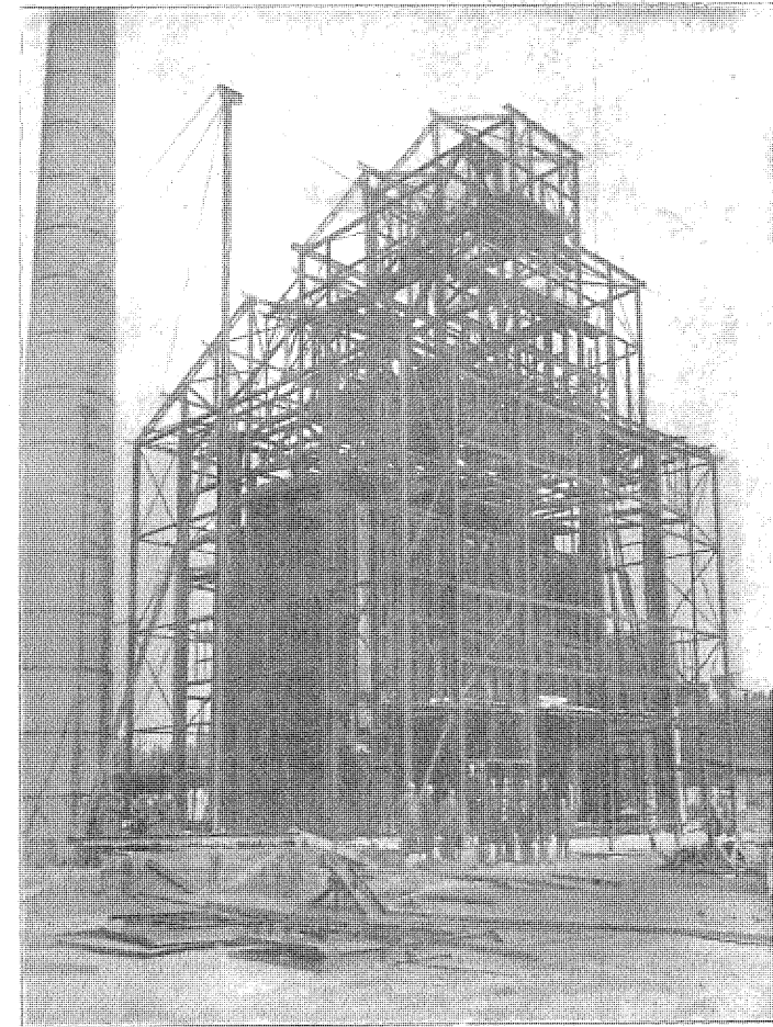
Nowa piecownia gazowni miejskiej w Łodzi w końcowej fazie robót. Do użytku oddana zostanie w początkach roku przyszłego. Roboty prowadzi inż. C. Kłobukowski i S-ka w Warszawie.
