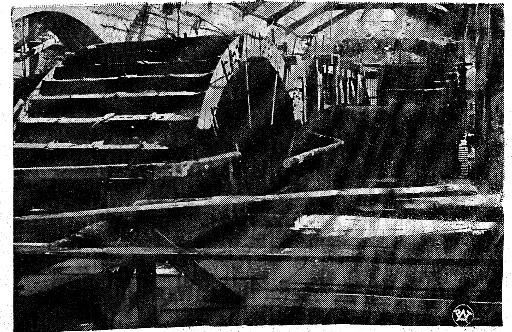
Koło wodne napędowe — ciekawa ilustracja z rezerwatu przechowującego w sobie wielką tradycję naszego rodzimego przemysłu metalurgicznego, który z odzyskaniem niepodległości rozrasta się w wielki ośrodek przemysłowy.
