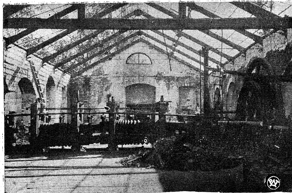
W ziemi kieleckiej, powiecie koneckim posiadamy bardzo ciekawy zabytek dawnej polskiej sztuki inżynierskiej — rezerwat techniczny. Rezerwat ten pochodzi z roku 1842, powstał za rządów księcia Lubbeckiego, ministra finansów Księstwa Warszawskiego.
