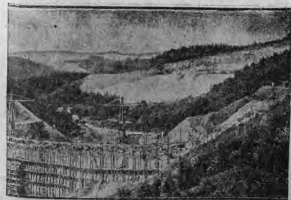
W okolicy miasta Lengenfeld (środkowe Niemcy) powstaje obecnie olbrzymi rozmiarów tama, która będzie największą tego rodzaju budowla w Europie. Na zdjęciu powyższem widzimy gigantyczną tamę w obecnym jej stadium.
