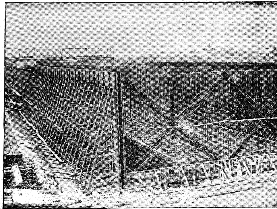
W Rotterdamie prowadzona jest budowa olbrzymiego tunelu pod rzeką Maas. Tunel ma stanowić arterię komunikacyjną dla samochodów, pojazdów i rowerzystów wówczas, gdy most zwodzony na rzece zostanie podniesiony w czasie przejścia wielkich okrętów.
