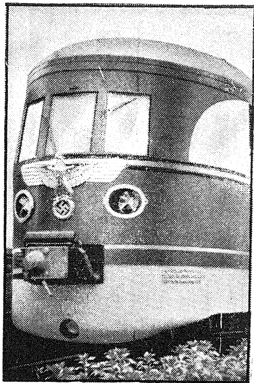
Niemcy uruchomili nowy motorowiec na trasie Berlin—Kolonja. Wagon-torpeda ma 2 motory Diesla, każdy po 600 koni mech i osiąga szybkość 160 km. na godz.
