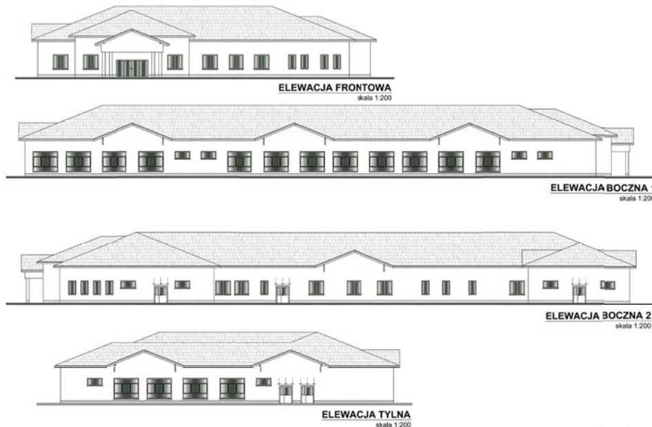
Koncepcje budynku żłobka miejskiego wraz z infrastrukturą towarzyszącą.
