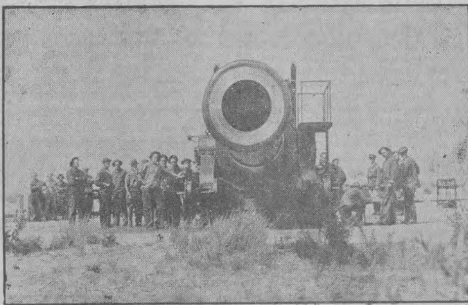
W amerykańskiej warowni nadmorskiej „Tilden” w stanie nowojorskim ustawiono imponujące działo dalekonośne, które wali 40 cm pociski o wadze 19 centnarów na odległość 25 km.
