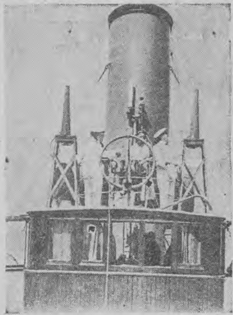
W ostatnich latach Marconi poświęcał się szczególnie badaniom fal ultrakrótkich i ich zastosowania do różnych celów. Laboratorium urządzono na pokładzie jachtu „Elektra”. Na zdjęciu Marconi na mostku kapitańskim „Elektry” podczas prób kierowania statkami na odległość. Po obu stronach mostu kierunkowe anteny nadawcze dla fal 40 centymetrowych.
