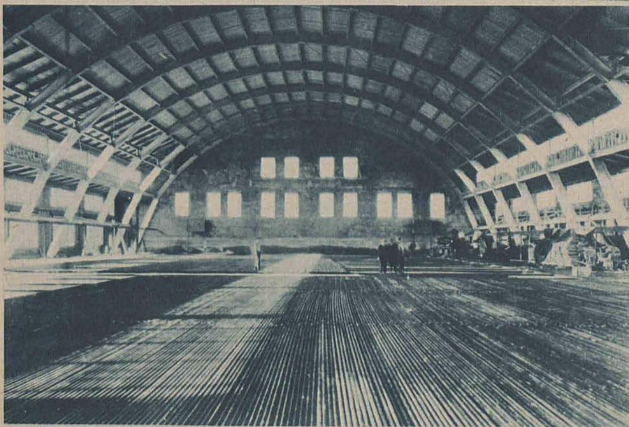
Z przygotowań do zawodów olimpijskich w Lake Placid. Hala w której odbędą się zawody hokejowe na lodzie.
