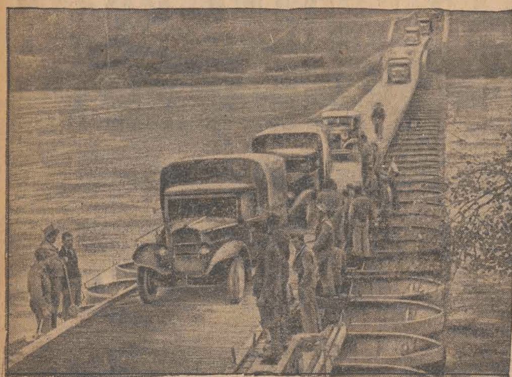
Most pontonowy zbudowany przez wojska powstańcze przez rzekę Ebro w miejscowości Mora.
