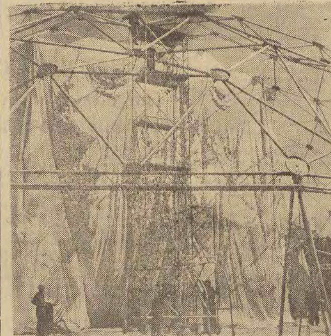
Na tereny targowe nadchodzą dalsze transporty z eksponatami wystawców zagranicznych. Trwają prace przy montażu lub renowacji pawilonów. Na zdjęciu: montaż pawilonu USA. Umocowywanie powłoki nylonowej na konstrukcji metalowej. CAF — fot. Urbanowicz
